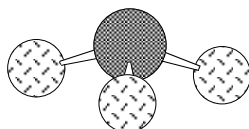
AX 3 E Pyramidal
