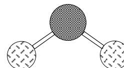
AX 2 E 2 Bent
